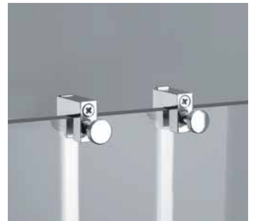
Particolare del fissaggio a vetro box doccia Magnification of fixing glass shower
